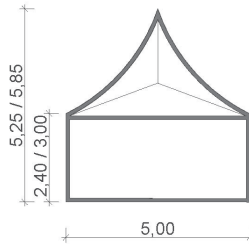
Seitenansicht
